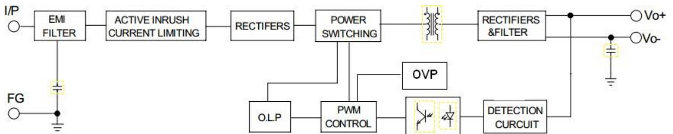
图表 1-2 内部电路结构框图
