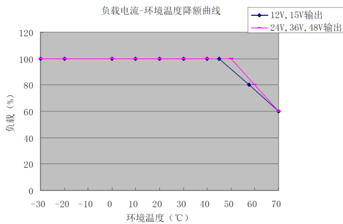
图表 3-1 负载电流-环境温度降额曲线
