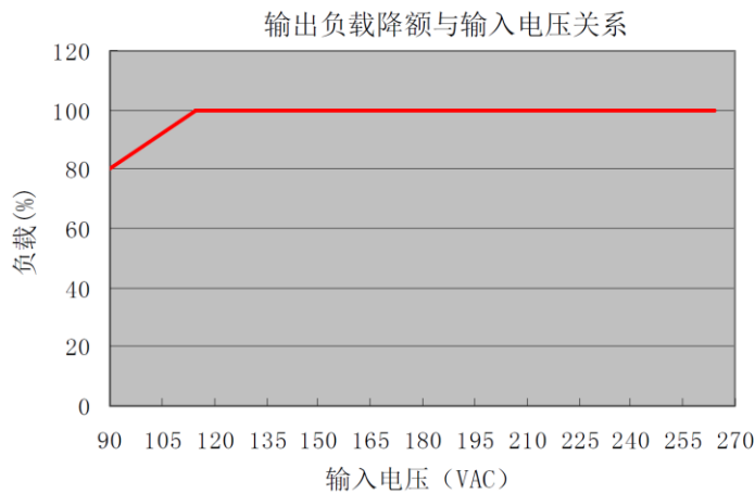
图表 3-2 输出负载特性曲线电流
